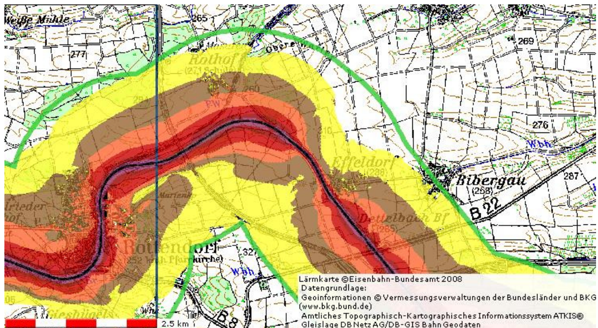
Bild 4: Isophonenkarte für die Nacht ( L_{Night} )
