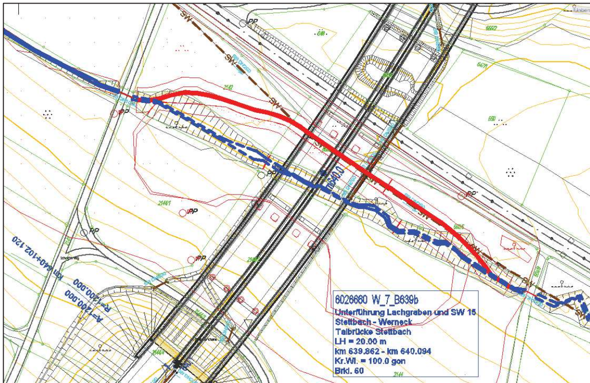
Abbildung 3-1 Unterführung des Lachgrabens (blau) – Vorfluter (rot)
