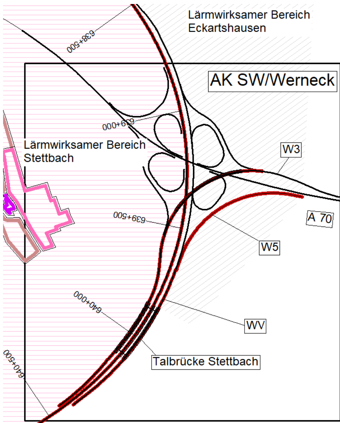
Bild 3: Systemskizze Fahrbahnbelag (k) – Detailausschnitt AK SW/Werneck
