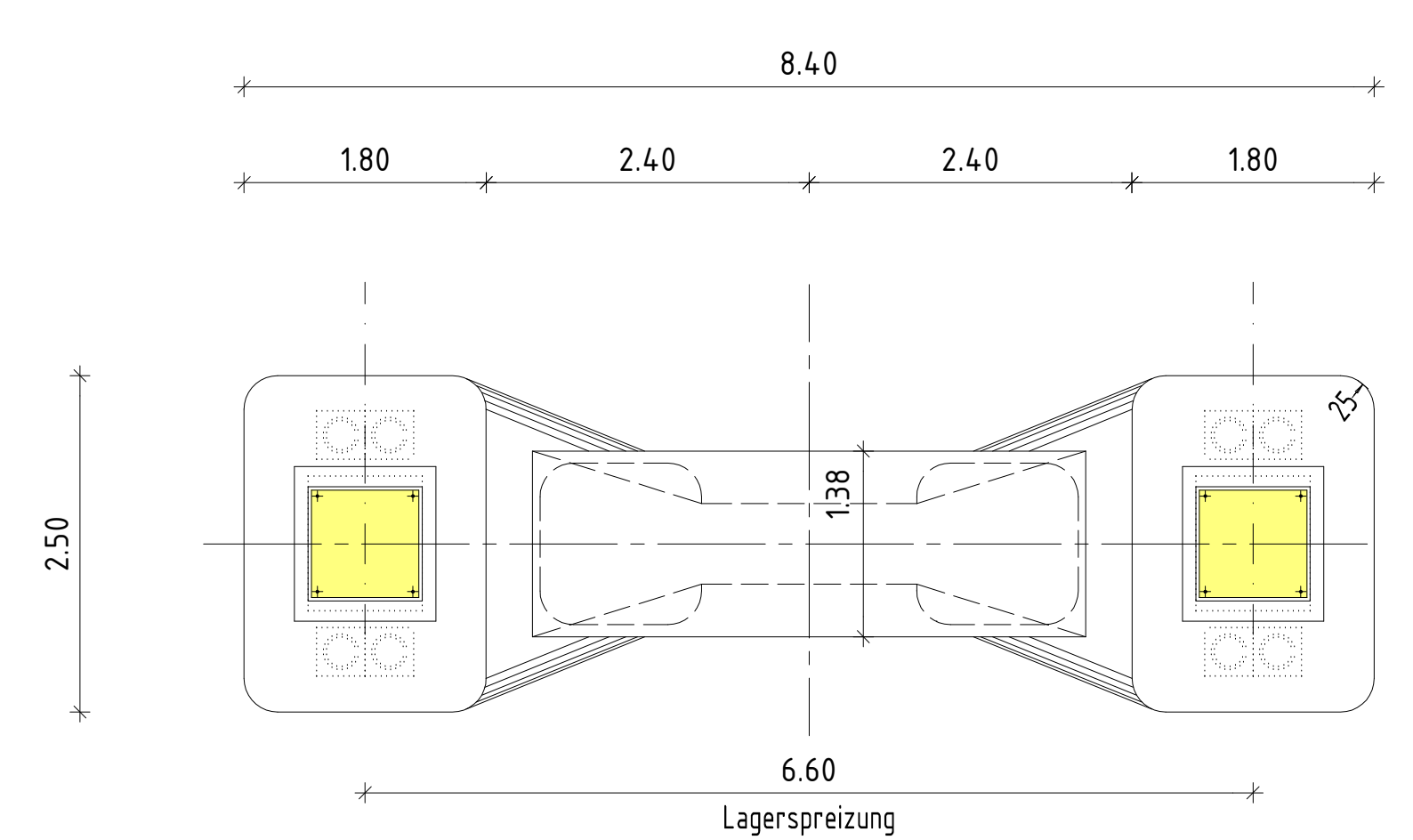
Draufsicht 1-1 Pfeilerkopf
