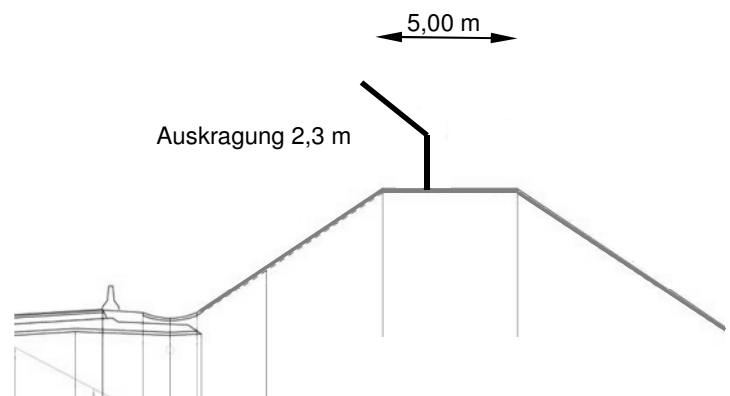
Querschnitt Planfeststellung 2014
