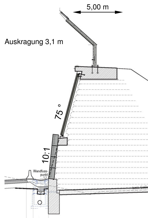
Querschnitt Planfeststellung 2014
