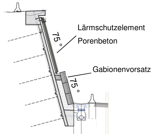
Querschnitt Planfeststellung 2014
