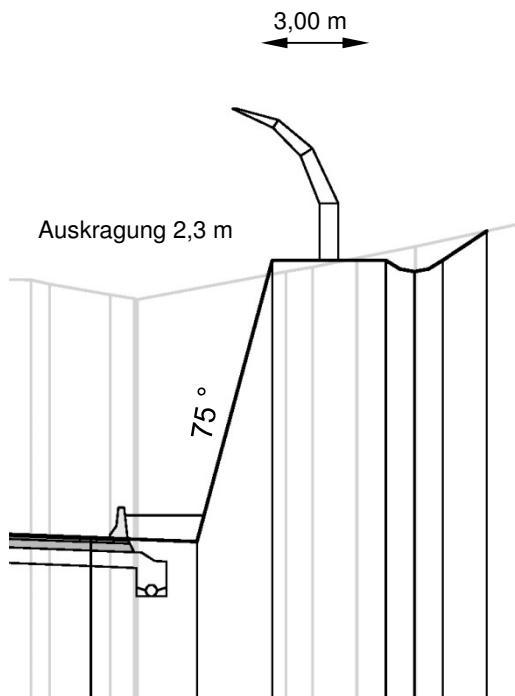
Querschnitt Planfeststellung 2008
