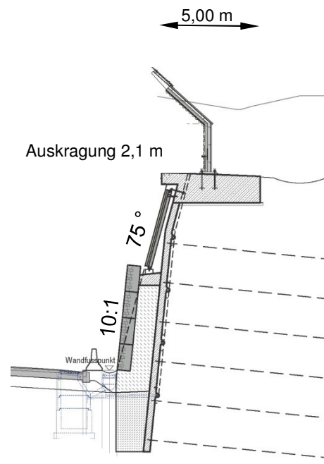
Querschnitt Planfeststellung 2014
