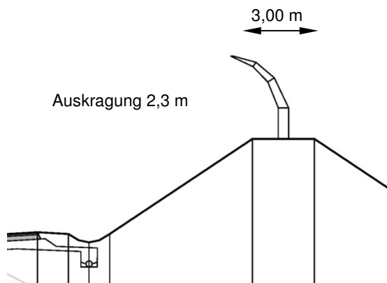
Querschnitt Planfeststellung 2008
