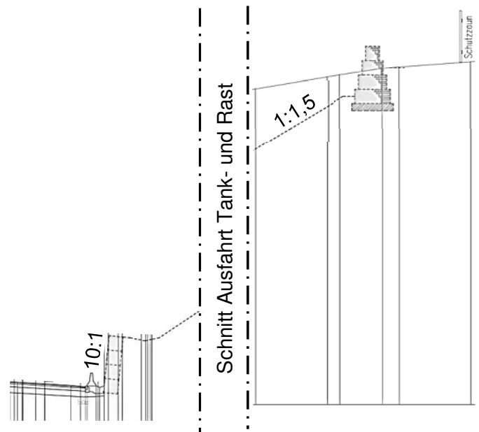
Querschnitt Planfeststellung 2014
