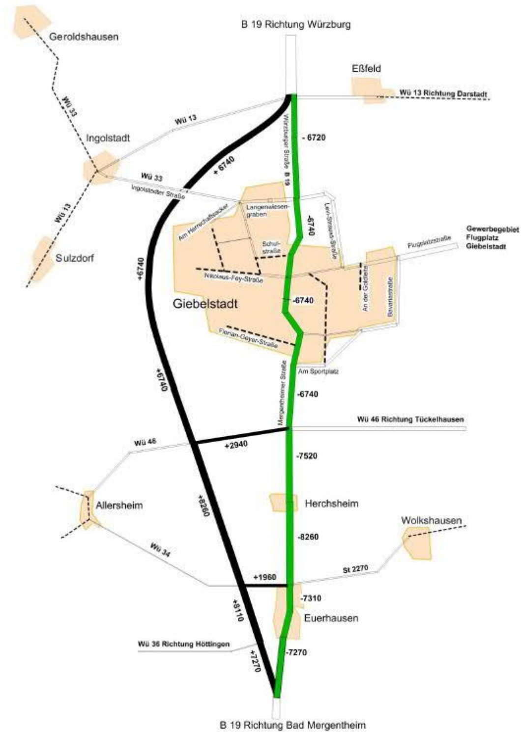
Abbildung 4: Belastungsveränderungen Prognoseverkehr 2035
