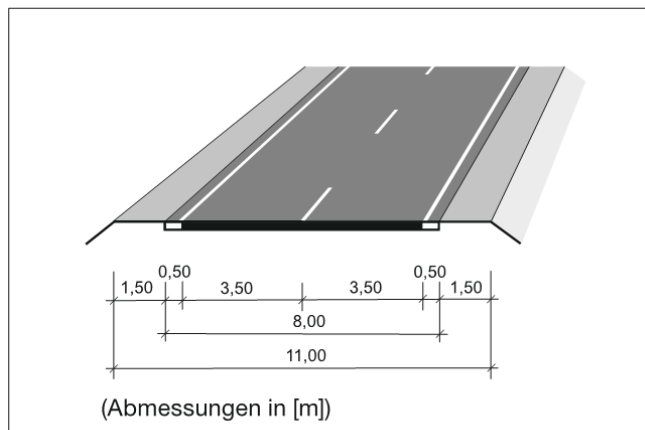
Bild 7: Regelquerschnitt RQ 11
