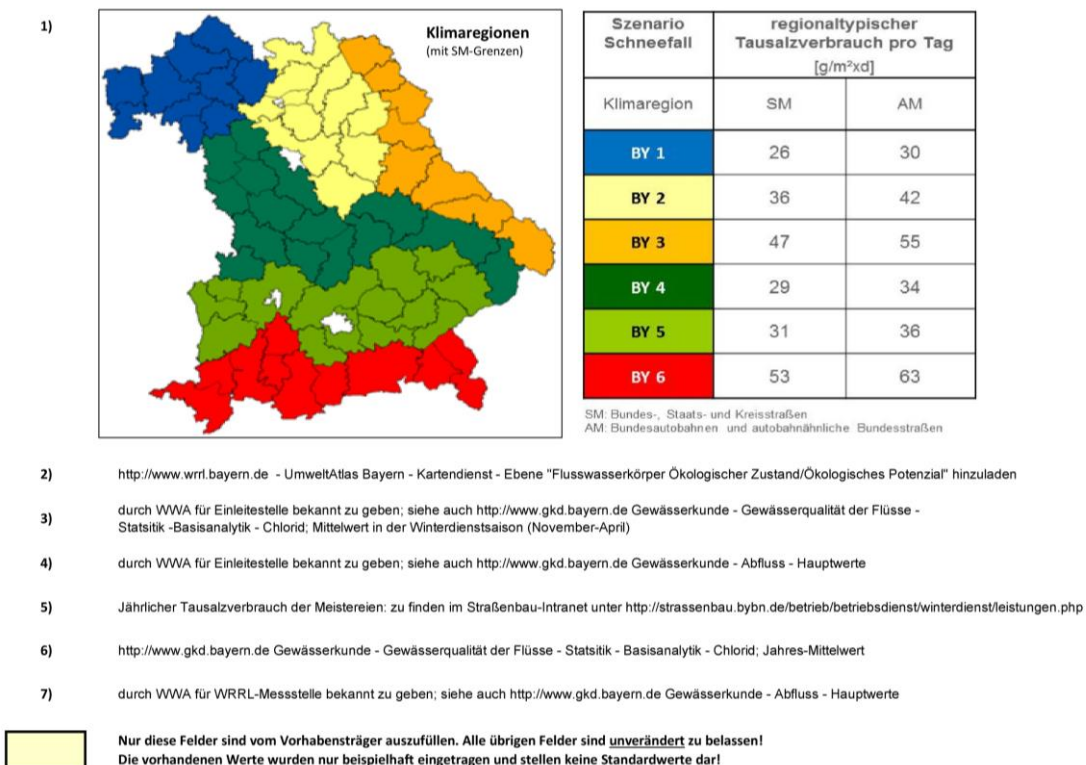
Abb. 7: Prüfformular zur Ermittlung des Jahresmittelwerts der Chloridkonzentration des Gewässers (Prognosezustand), Teil 2 3
