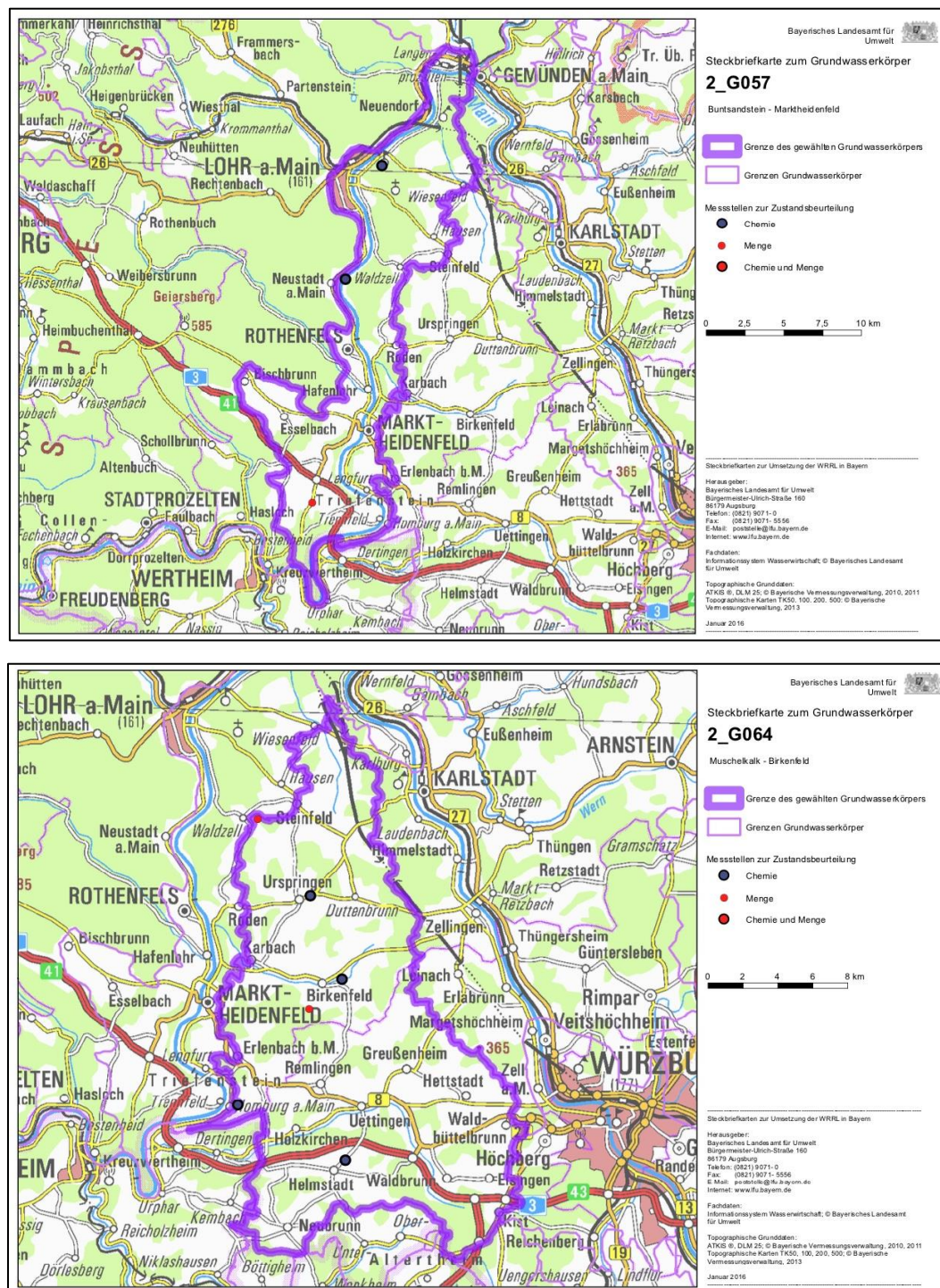
Abb. 1: Grundwasserkörper (Steckbriefkarten des BayLfU, Datenquelle Umweltatlas Bayern, Gewässerbewirtschaftung)
