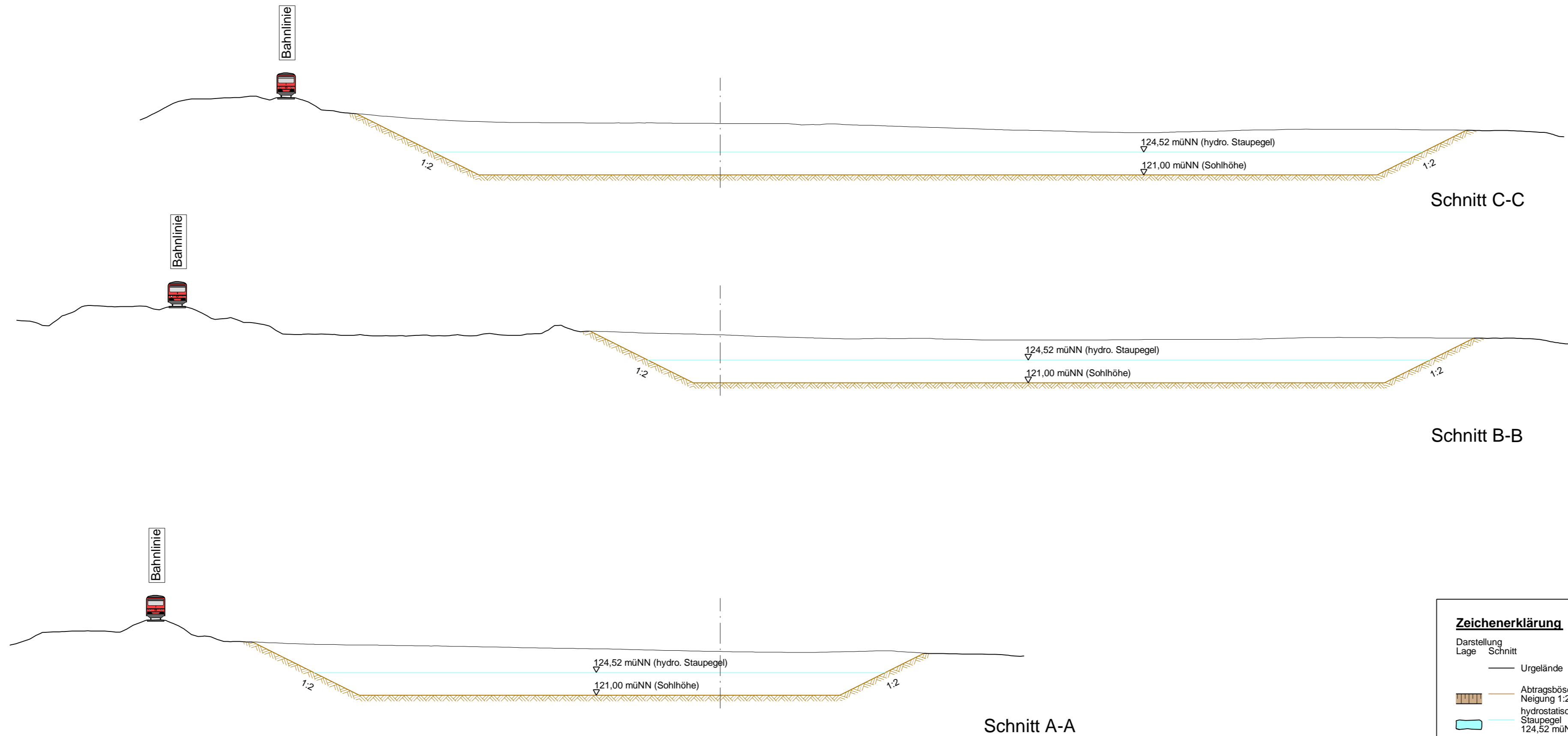
Querschnitte M 1:500
